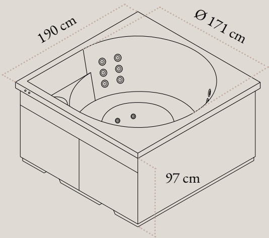
DROP COMPACT 190 x 190 CM (Vuolle Compact sur l’image)
