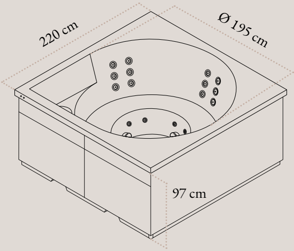
DROP SPAS 220 x 220 CM (Vuolle sur l’image)
