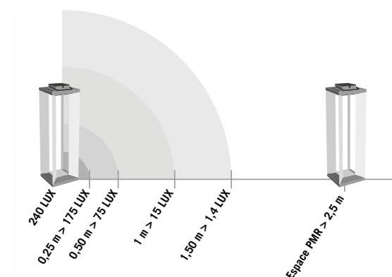
IMPLANTATION LUX /DISTANCE TEST RÉALISÉ AVEC UNE LAMPE TECKA98 500 LM
