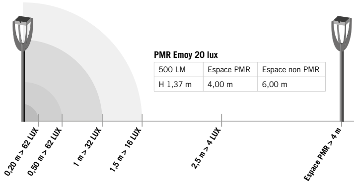
IMPLANTATION LUX /DISTANCE TEST RÉALISÉ AVEC UNE TORCHE TINK300 OPTION 500 LM
